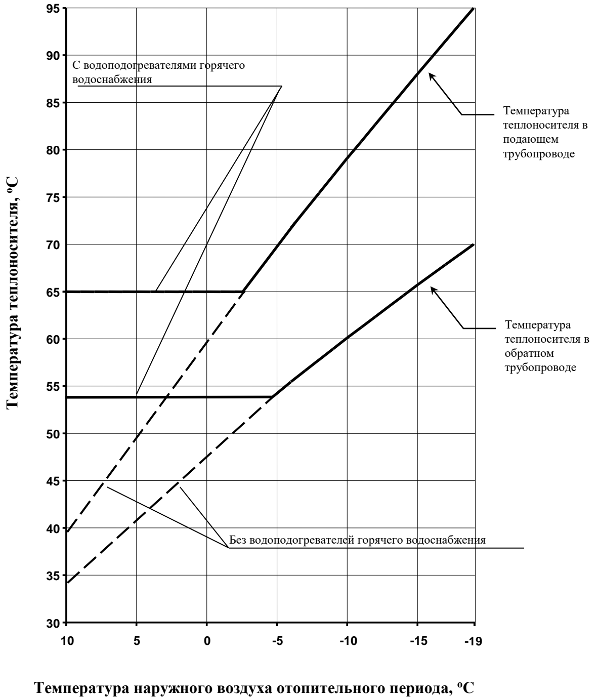
Температурный график качественного регулирования теплоносителя (95 - 70 °С)
